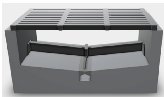
Unterflurschieber mit Quergefälle unter Spaltenboden (Quelle: Kuratorium für Technik und Bauwesen in der Landwirtschaft)
