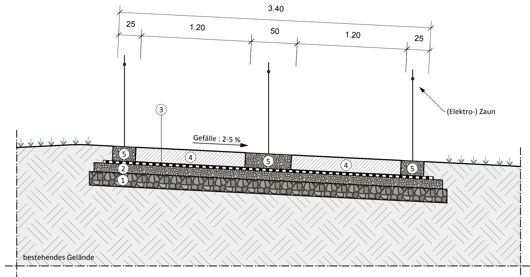
Querschnitt
