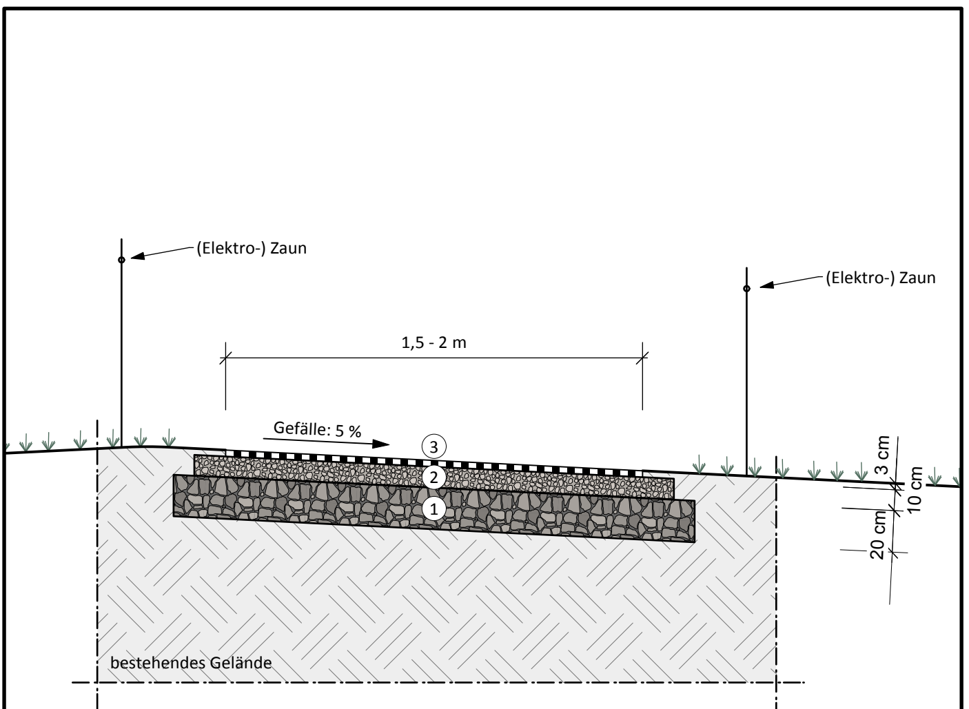
Querschnitt
